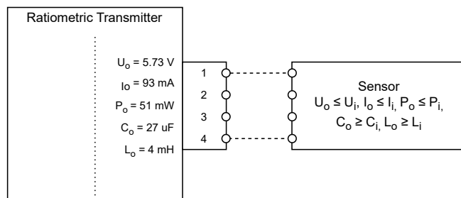
Figure 6.1: Valeurs limites de sécurité intrinsèques
