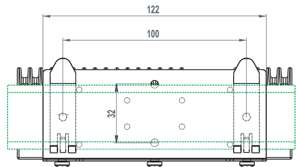
Fig. 4.21: L-bracket
